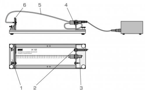
IA120 princíp fungovania priemyselných senzorov
